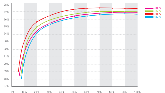
Growatt 6000UE Wirkungsgrad
